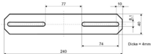
Maße Universaltraverse
